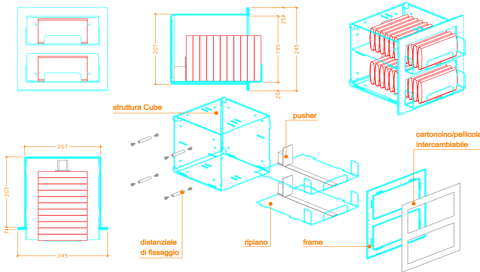
Particolari tecnici del modello orizzontale Technical details for the horizontal model
