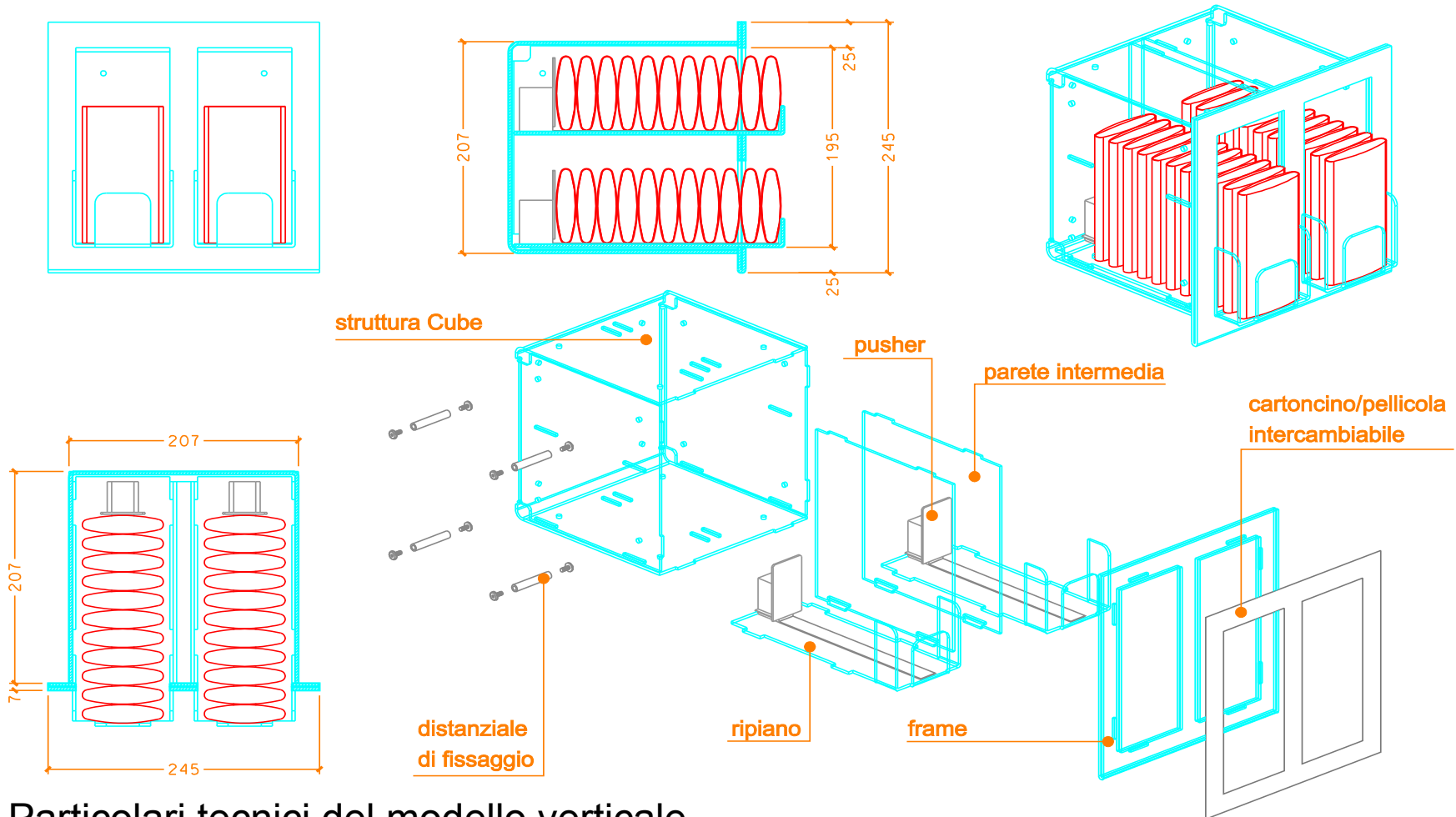
Particolari tecnici del modello verticale Technical details for the vertical model
